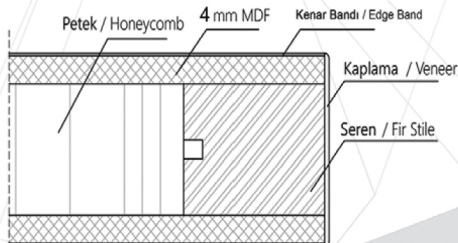
Kaplamalı Kapı Kanadı Kesiti Veneered Door Leaf Section
